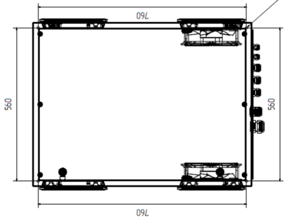
Рис. 5. Установочные размеры*
