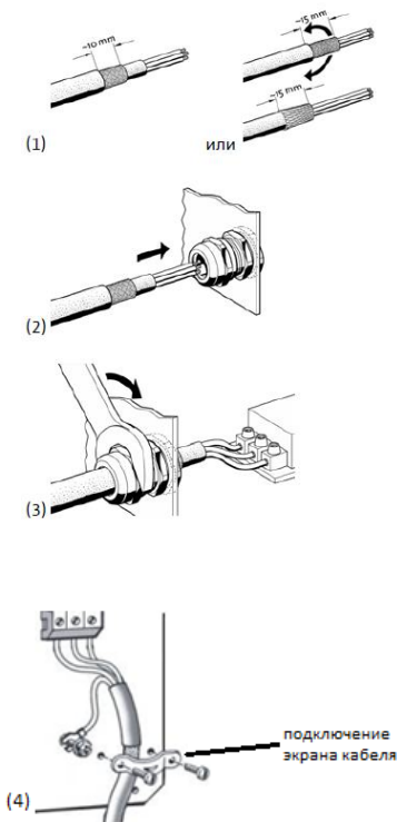
Рис. 15. Подключение кабеля насоса к прибору управления.
